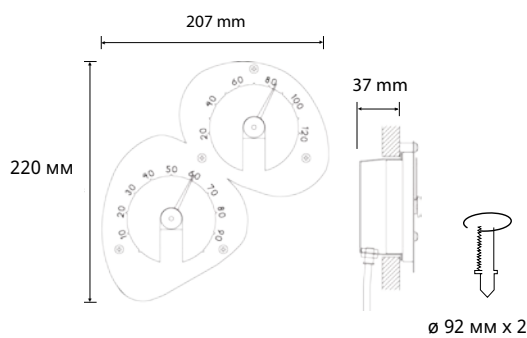
ТЕРМОМЕТР-ГИГРОМЕТР Артикул 1545822
