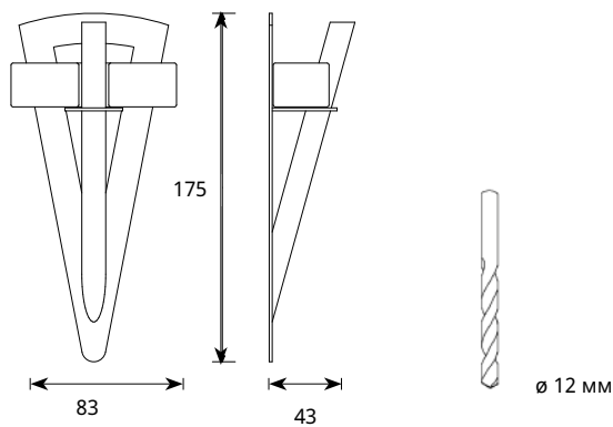
TL-100 Артикул 1545801
