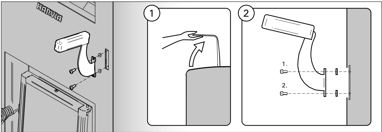
Рисунок 13. Установка рукояток
