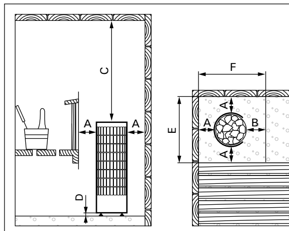
Рисунок 4. Расположение и безопасные расстояния (все размеры приведены в миллиметрах)
