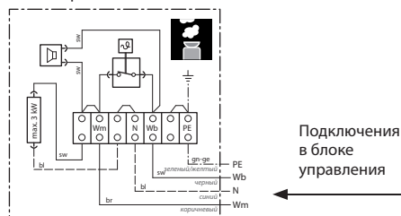
Испаритель
