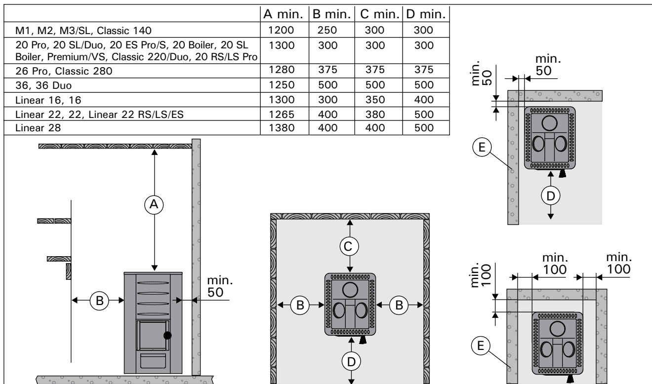
Рисунок 7. Безопасные расстояния (все размеры приведены в миллиметрах) Joonis 7. Ohutuskauused (kõik mõõtmised millimeetrites)
