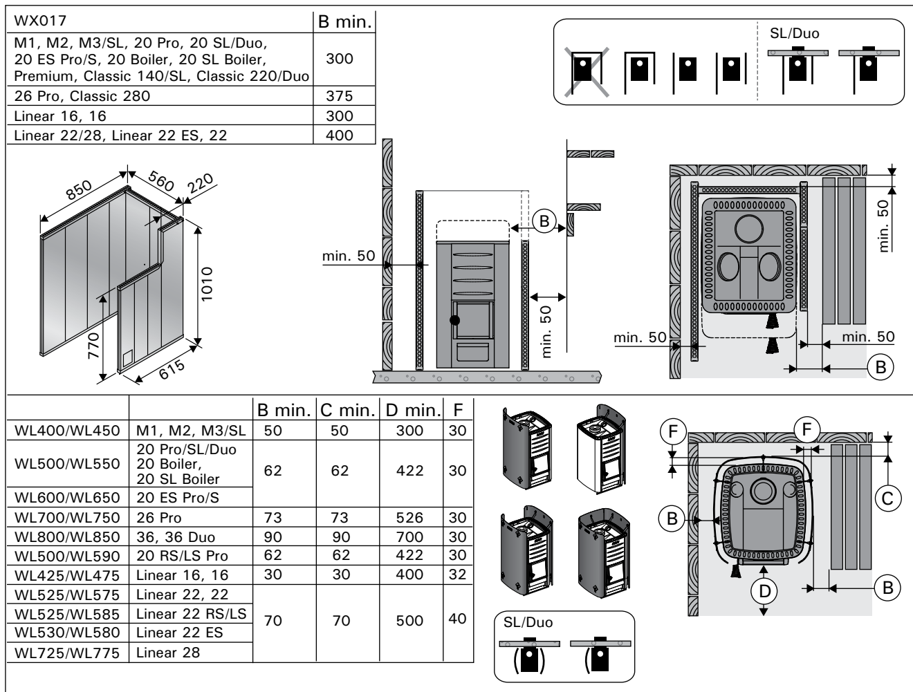
Рисунок 8. Безопасные расстояния с защитными ограждениями (все размеры приведены в миллиметрах) Joonis 8. Ohutuskaukus koos kaitseseinaga (kõik mõõtmised millimeetrites)
